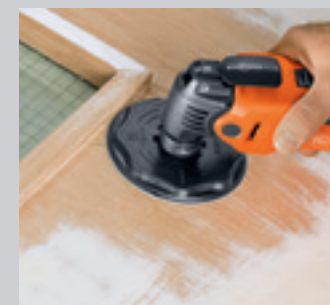
Het grote ronde schuurplateau vervangt extra schuurmachines zoals excenter- of vlakschuurmachines.
